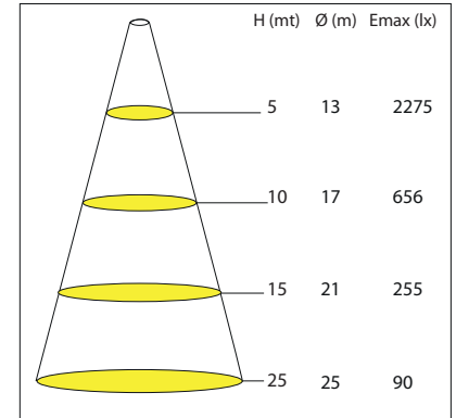
LPR20.600 600W 4000K 60DG 230VAC IP66
