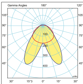
Double Asimetrik
