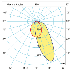
Asimetrik
